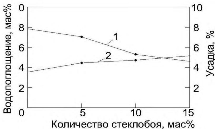
Рис. 2 – Влияние количества стеклобоя на водопоглощение (1) и усадку (2) при температуре 1100 °C
