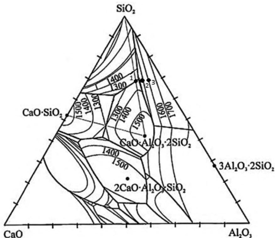
Рис. 1 – Расположение составов в системе \text{CaO}-\text{Al}_2\text{O}_3-\text{SiO}_2
