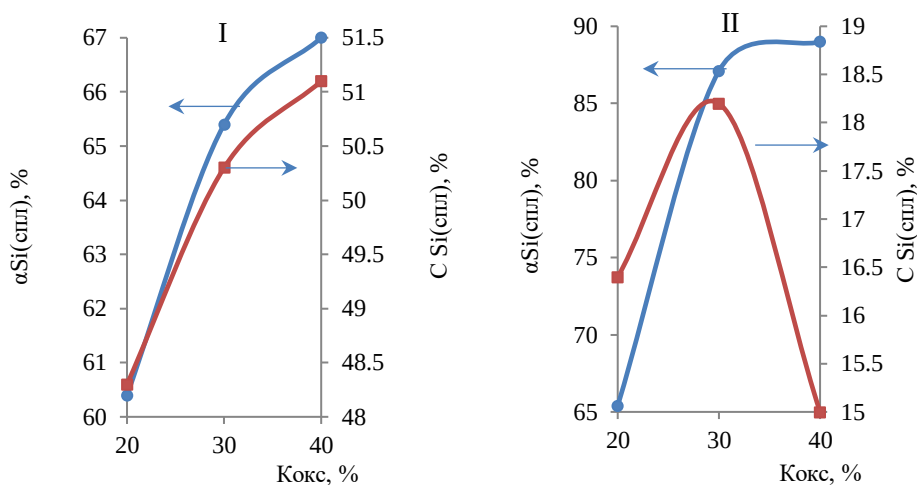
Рисунок 2 – Влияние количества кокса и стальной стружки на степень извлечения и концентрацию кремния в сплаве
