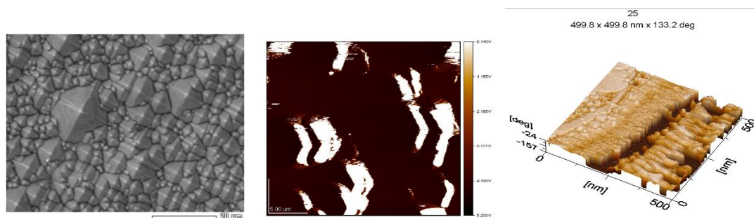
Рисунок 1 – АСМ-изображения образца без покрытия: (а) оптическая микроскопия; (б) 25 \times 25 мкм (режим топографии), (в) 500 \times 500 нм (фазовый режим)
