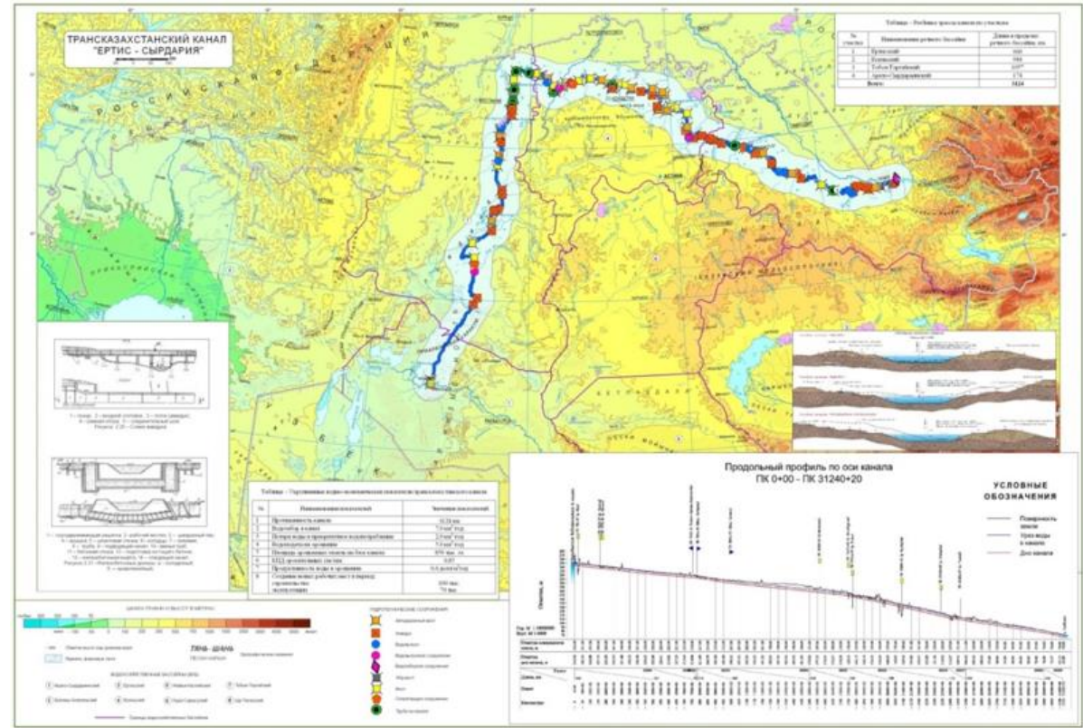
Рисунок 7 – Трансказахстанский канал
