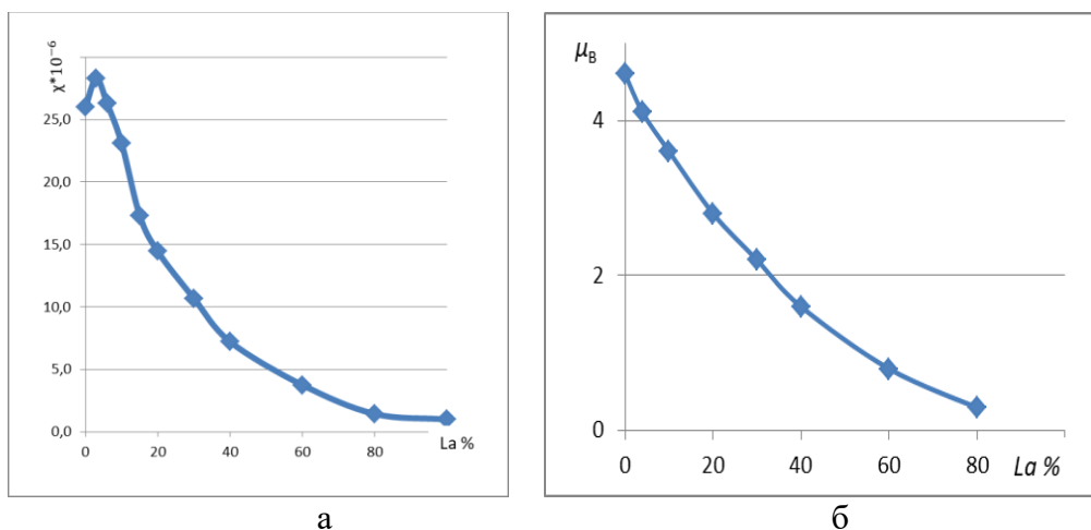
Рисунок 1 – Изотермы \chi (а) и концентрационные зависимости \mu_{\text{эф}} (б) сплавов железо-лантан в жидком состоянии
