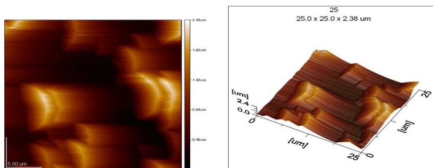
Рисунок 2 – АСМ-изображения образца с 25 слоями покрытия, масштаб сканирования – 25 \times 25 мкм: а – топографический режим; б – фазовый режим
