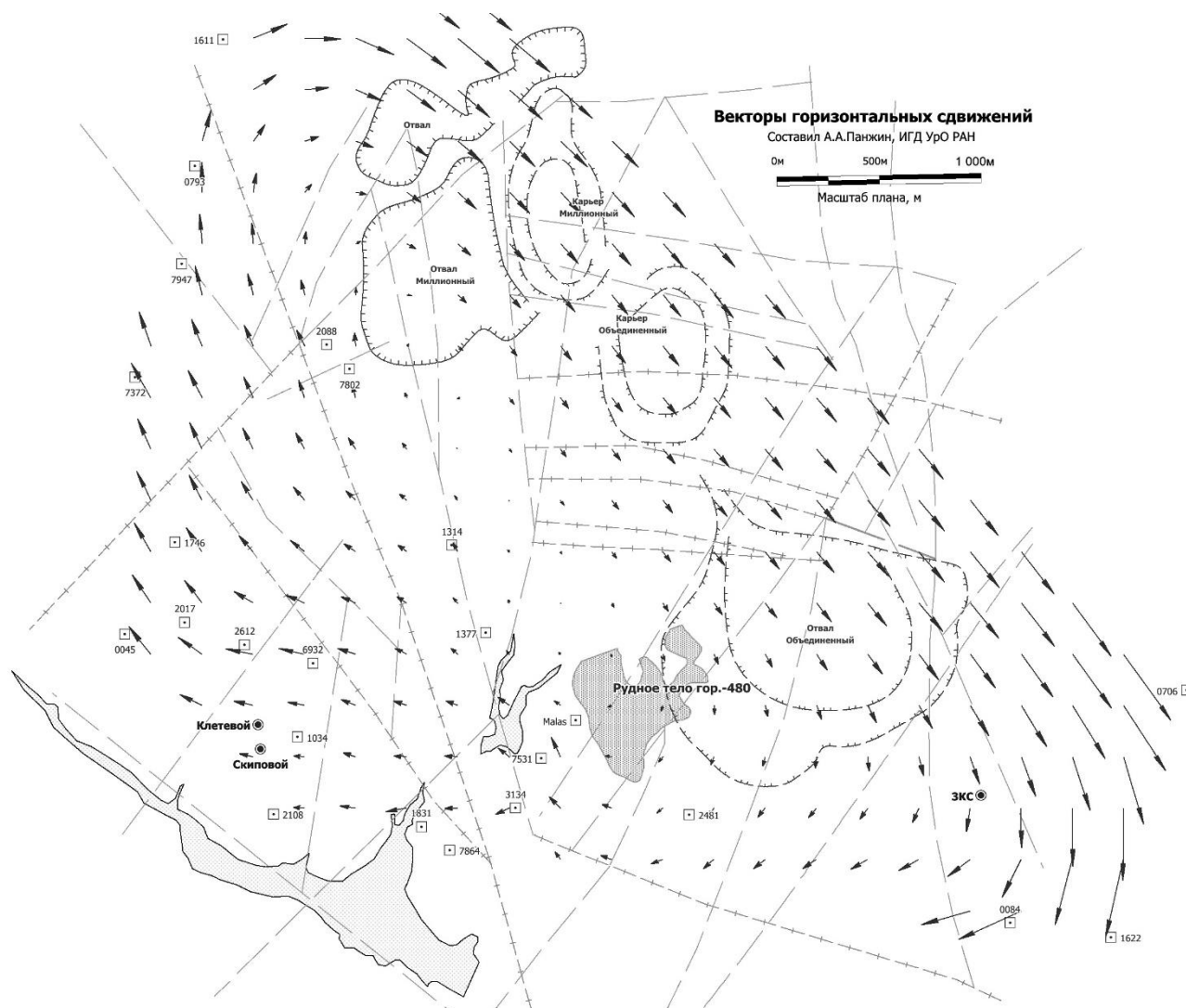
Рисунок 2 – Векторы горизонтальных сдвижений
