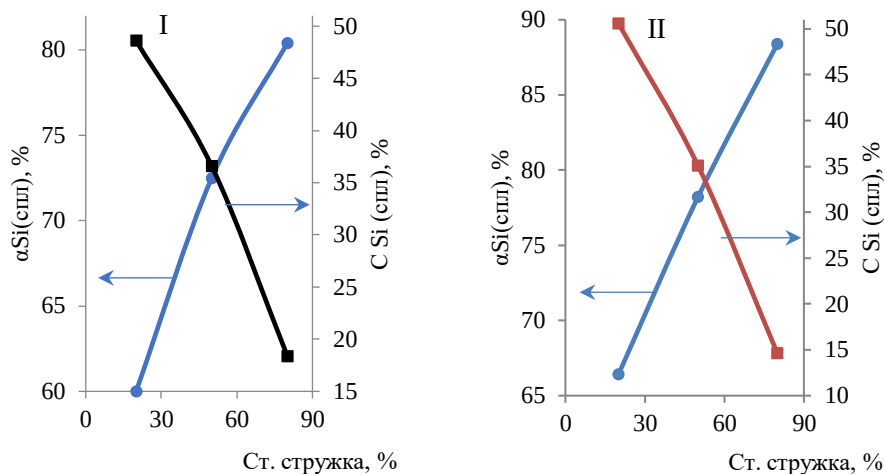
Рисунок 1 – Влияние количества стальной стружки и кокса на степень извлечения и концентрацию кремния в сплаве
