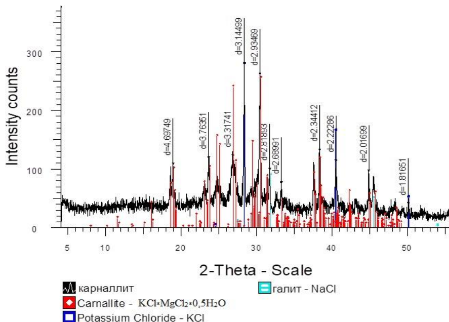
Рисунок 1 – Дифрактограмма карналлита
